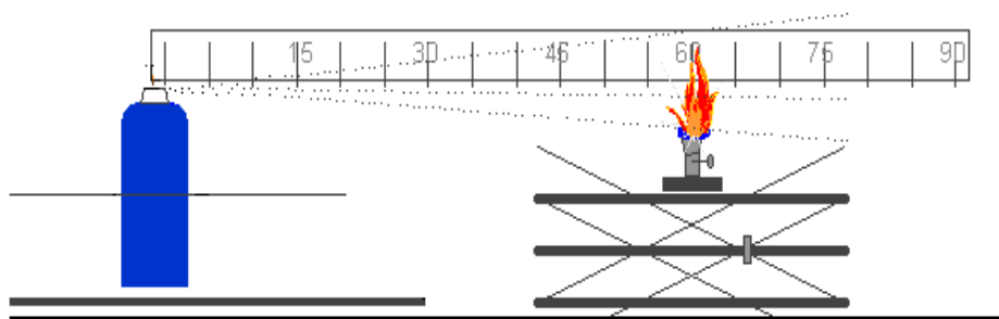
Figure 31.4.1 : Installation pour l'épreuve d'inflammation à distance
